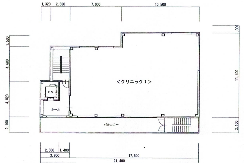
2階平面図 1/200
