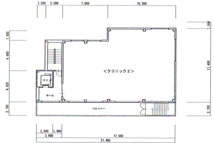
3階平面図 1/200
