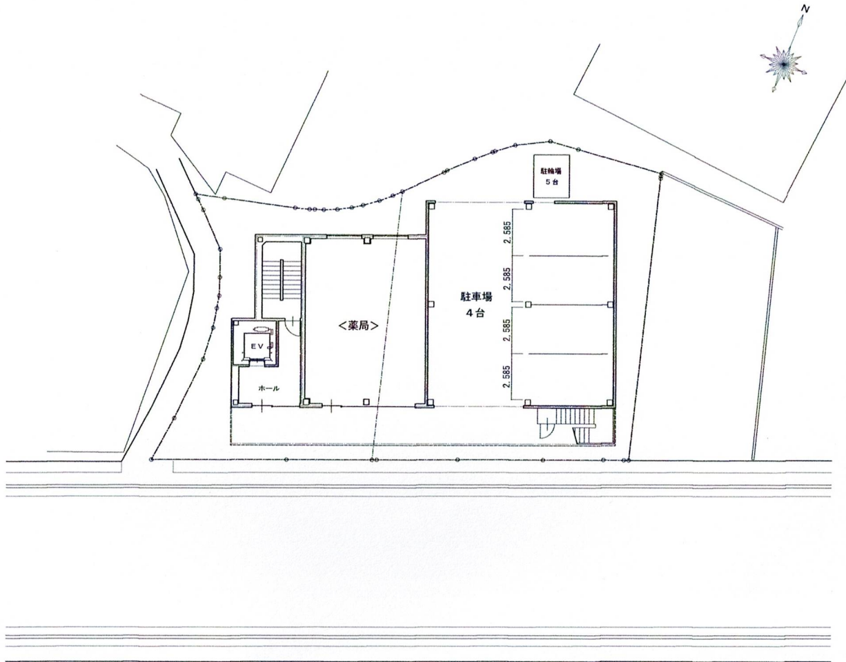
1階平面図 1/200
